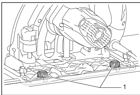
► 1. Регулировочные винты
