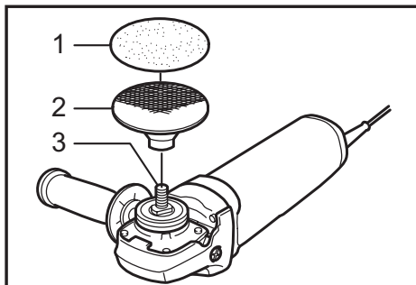
▶ 1. Абразивный диск 2. Опорная пластина 3. Шпиндель
