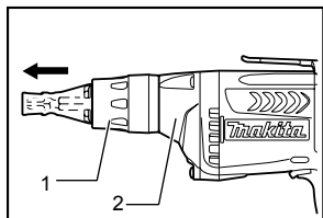
1. Стопорное кольцо 2. Корпус редуктора
